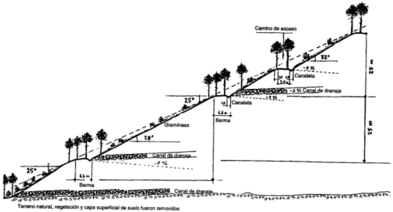
Figura 3 - Sección esquemática de una pila de estériles
