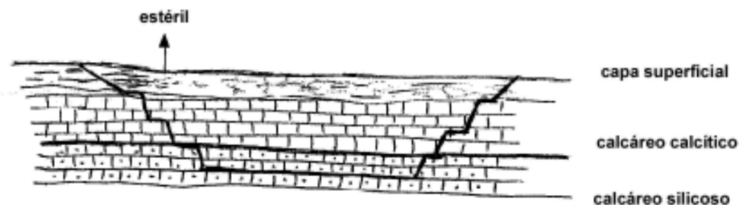
Figura 2 - Representación esquemática del perfil de una cava de calcáreo sedimentario donde las capas tienen diferentes composiciones químicas: dependiendo del uso de la minera, algunas capas pueden ser consideradas como estériles, así como el suelo de alteración, llamado capa superficial del yacimiento.
