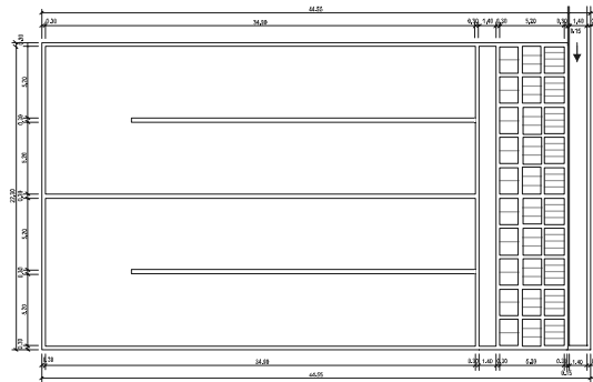
Figura 3-4. Sistema convencional antiguo
