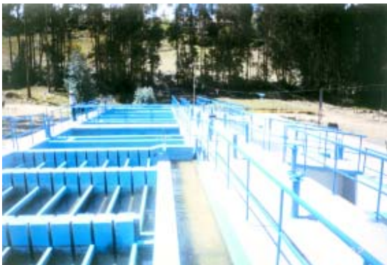
Figura 3-7. Planta de tecnología apropiada de 120 L/s (3)
