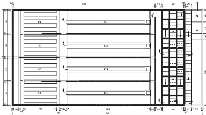
Figura 3-5. Sistema convencional optimizado
